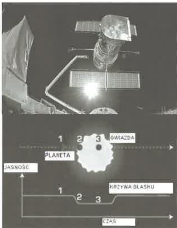
Schemat przedstawiający kolejne fazy tranzytu planety pozasłonecznej.
