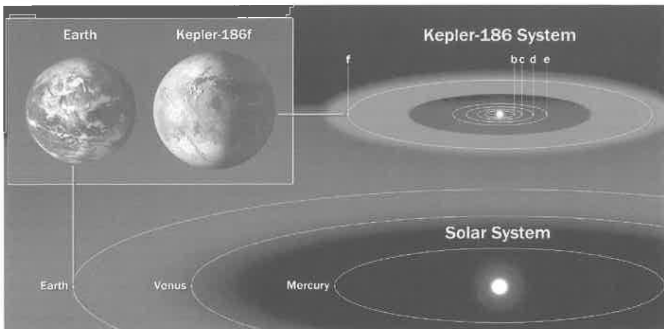
System Kepler-186 i wewnętrzny Układ Słoneczny
