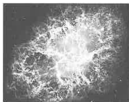
Mgławica Krab — najświeższy obraz pozostałości po wybuchu supernowej z roku 1054, uzyskany aparatem FORS w ognisku 8,2 m teleskopu zespołu VLT obserwatorium ESO na górze Paranal w Chile.
