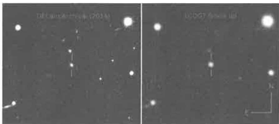
Obrazy w fałszywych kolorach pokazujący galaktykę przed eksplozją ASASSN - 15lh wykonany przez Dark Energy Camera (z lewej) i supernowej przez sieć 1-metrowych teleskopów w Las Cumbres Observatory Global Telescope Network (z prawej)
